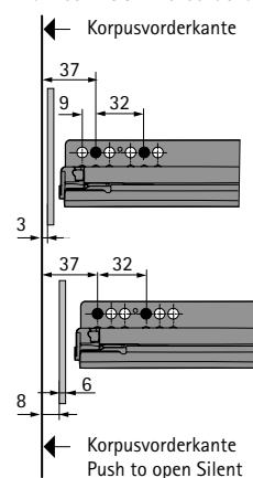
AvanTech YOU Innenschubkasten / Innenauszug
