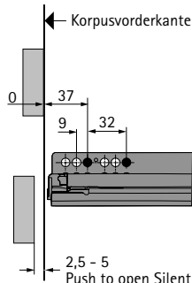
AvanTech YOU Schubkasten / Frontauszug
