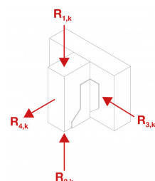
Vollausnagelung
