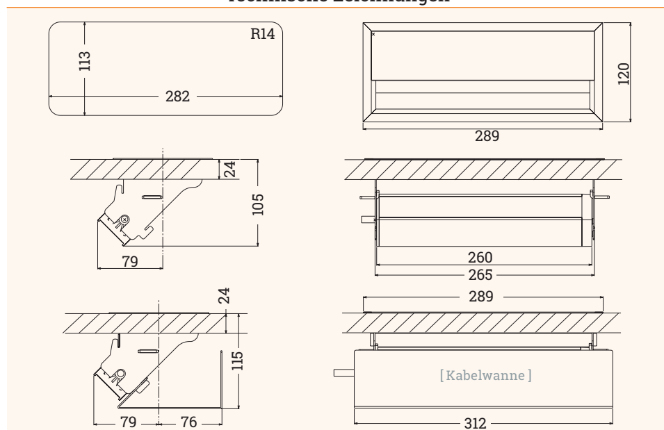
Technische Zeichnungen
