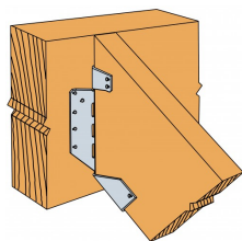
Geneigte Verbindung
