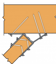
LSSU Befestigung
