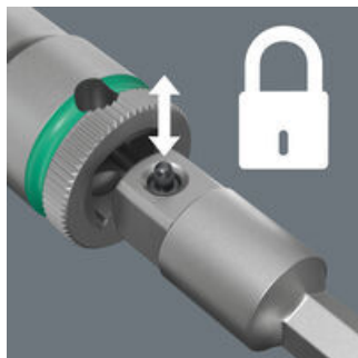
Die federnde Kugel auf dem Vierkant greift in die Bohrung des Steckschlüsseinsatzes und sichert so den Steckschlüsseinsatz auf dem Verbindungsteil.
