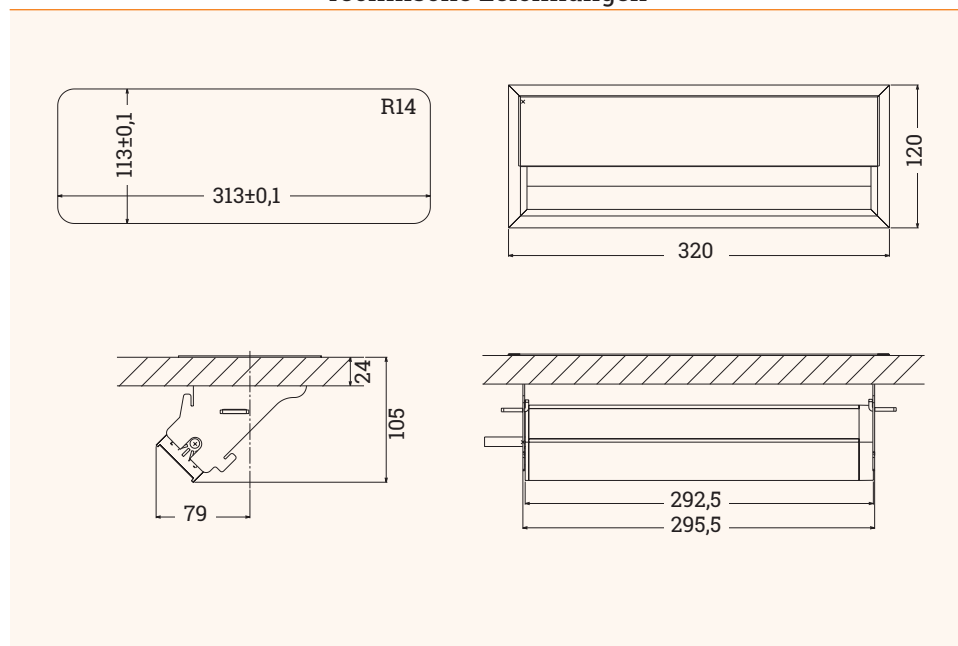
Technische Zeichnungen
