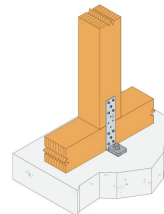
Fig. 3 : Installation innenliegend
