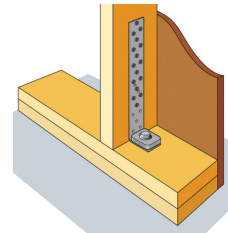
Fig. 3 : Installation innenliegend
