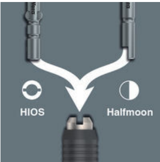
Kombinationsbithalter für Bits mit Halfmoon und HIOS-Antrieb.
