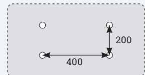
Position: Bohrlöcher im AKUSTIX Element
