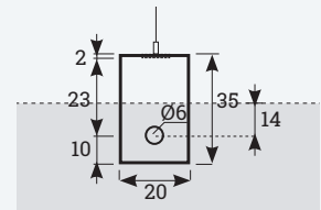
Position: Bohrlöcher im AKUSTIX Element
